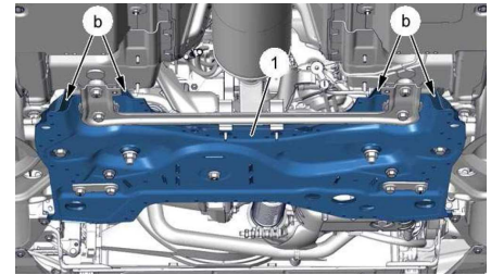
フロントサブフレーム
